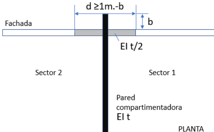
Figura 2.4: Compartimentación con fachada plana ( \alpha=180^\circ ) y saliente vertical.
